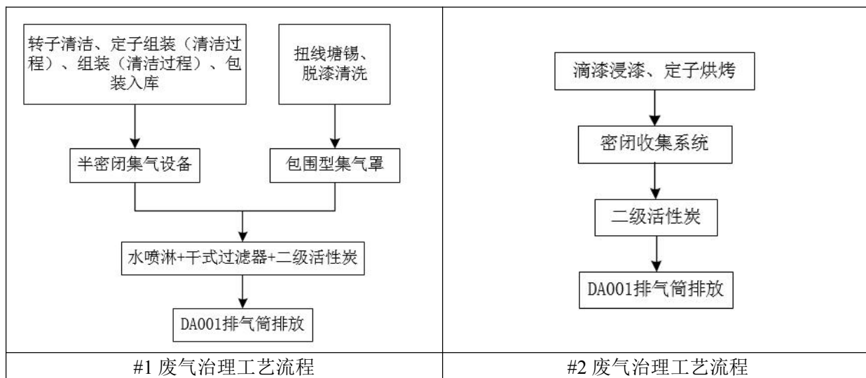
图 4-1 项目废气治理工艺流程图
