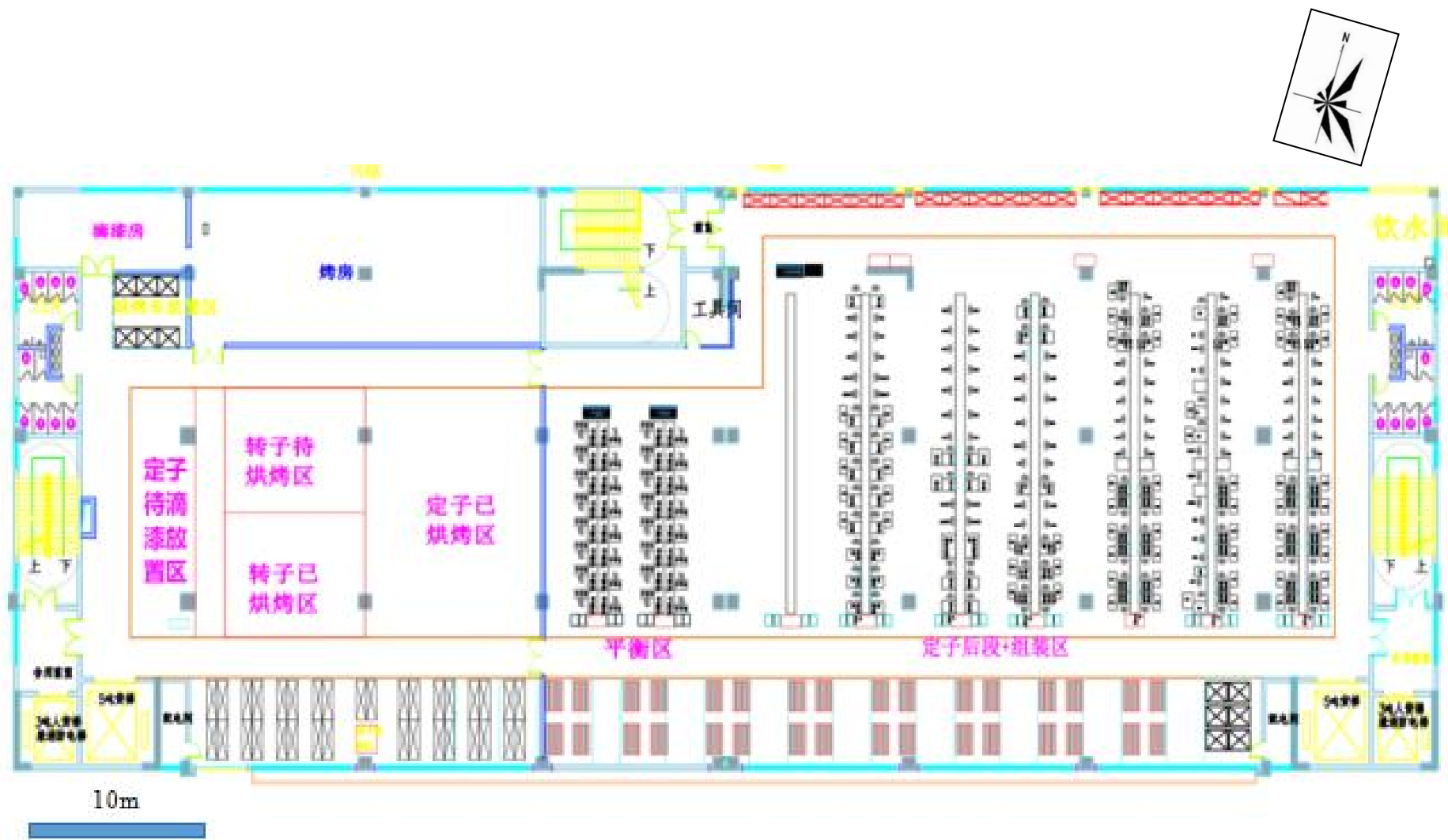
图 3-7 A 栋厂房车间平面布置图（4 楼）
