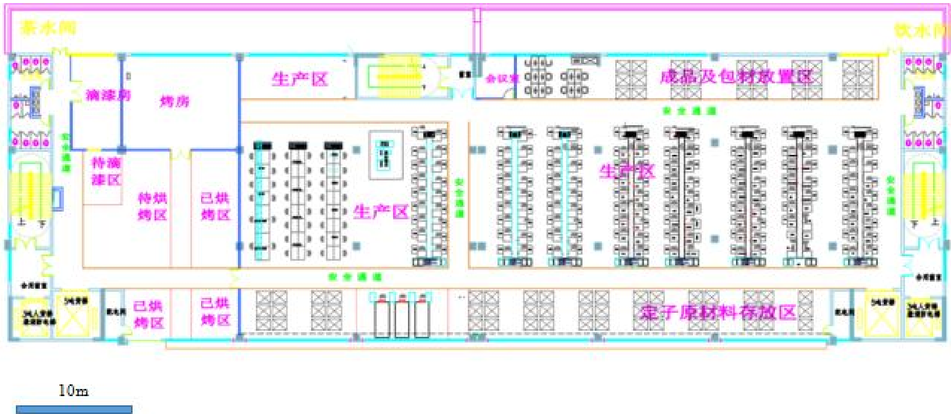
图 3-8 A 栋厂房车间平面布置图 (5 楼)
