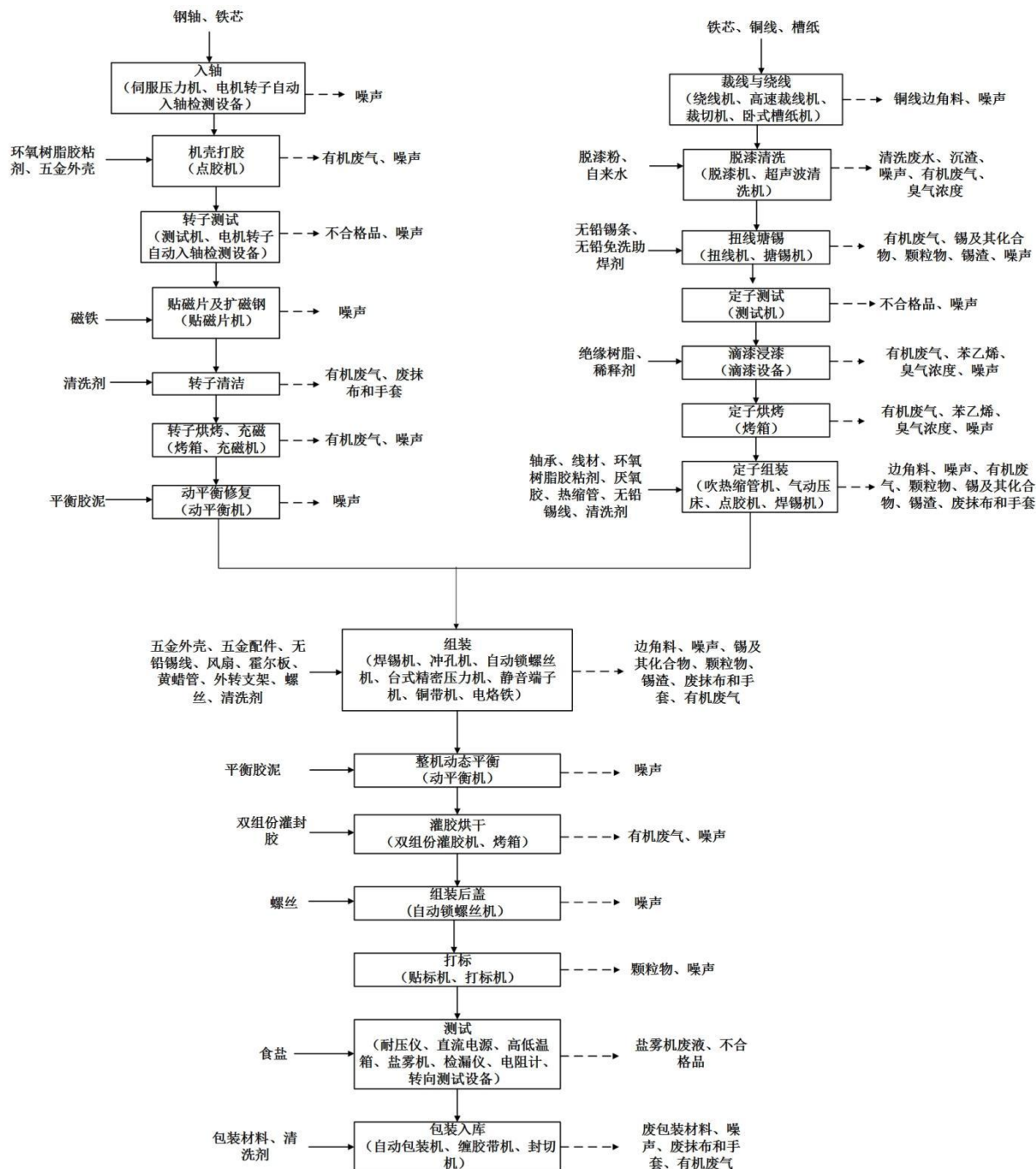
图 3-13 无刷电机工艺流程及产污环节图
