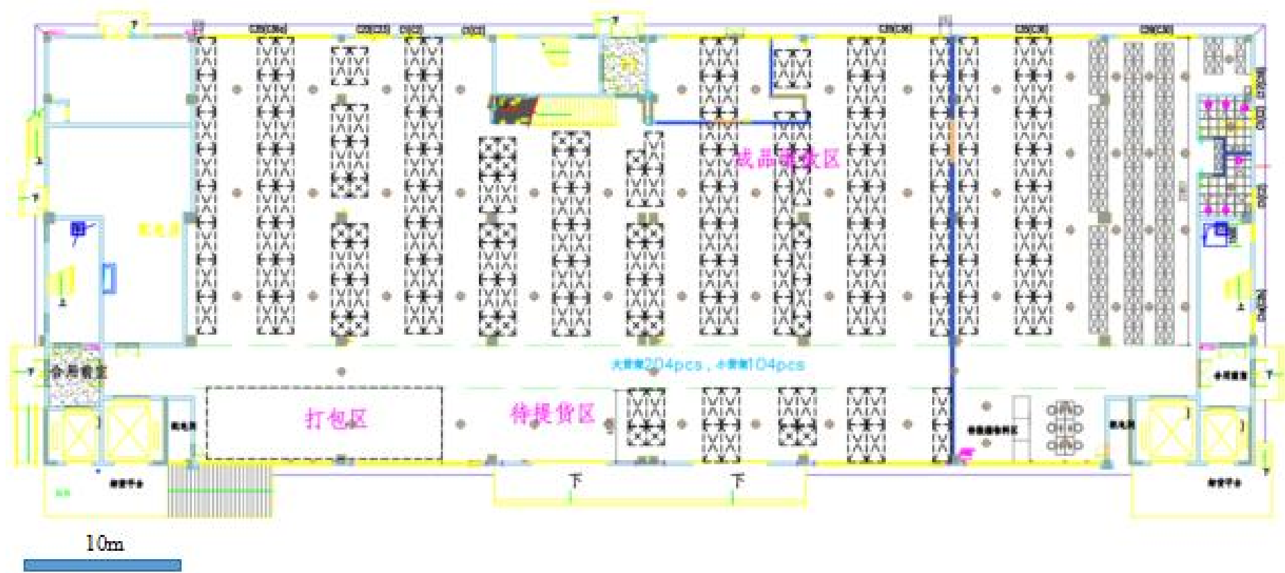
图 3-4 A 栋厂房车间平面布置图（1 楼）
