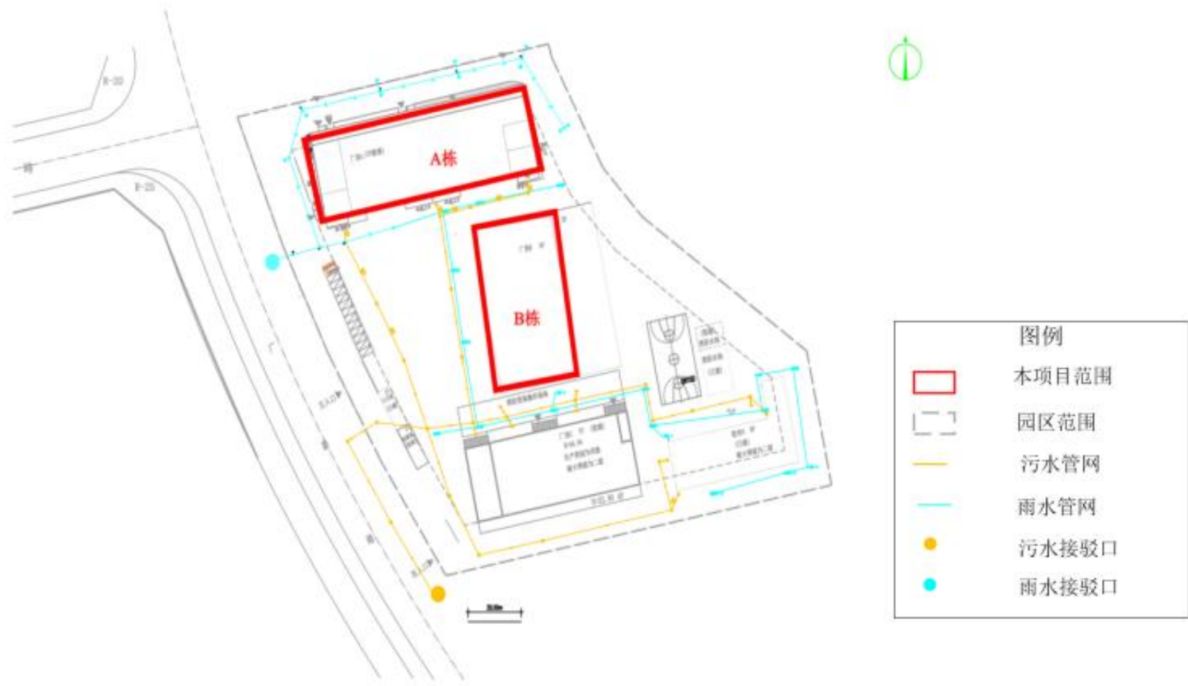
图 3-12 项目厂区雨污分流图
