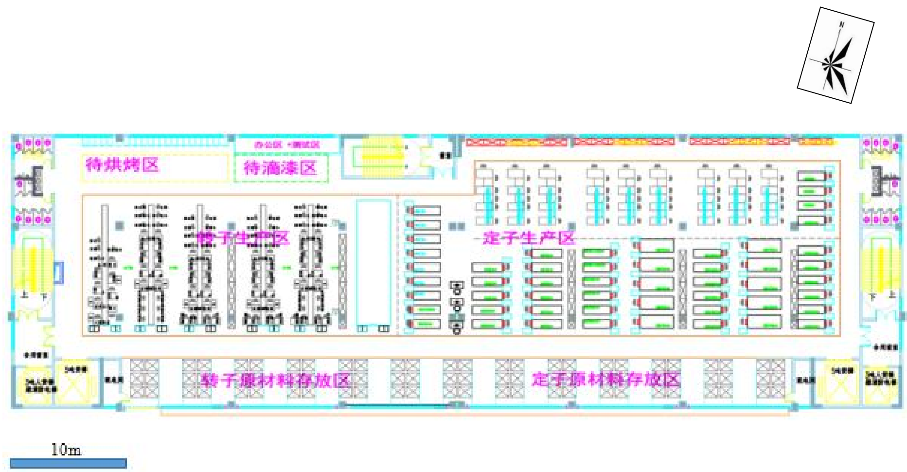
图 3-9 A 栋厂房车间平面布置图（6 楼）
