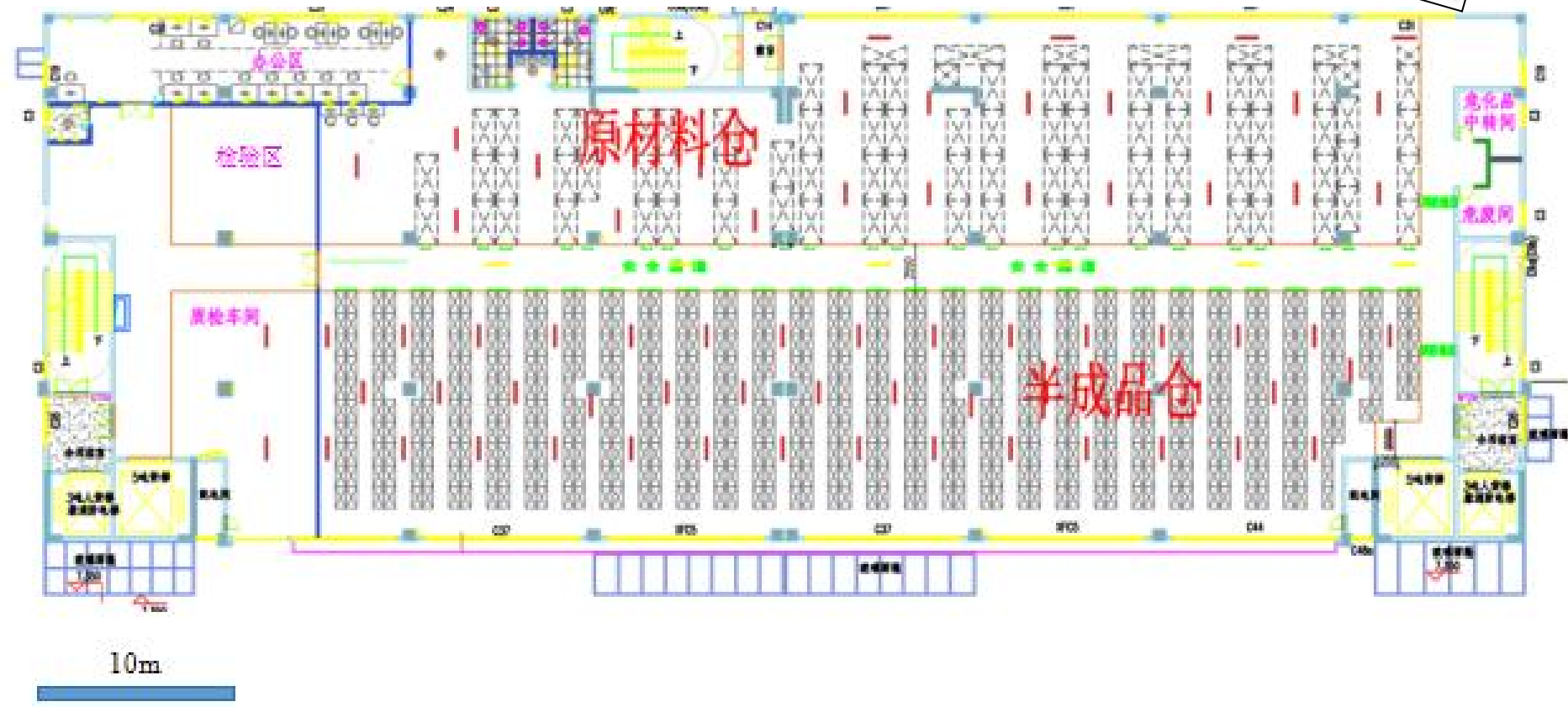
图 3-5 A 栋厂房车间平面布置图（2 楼）
