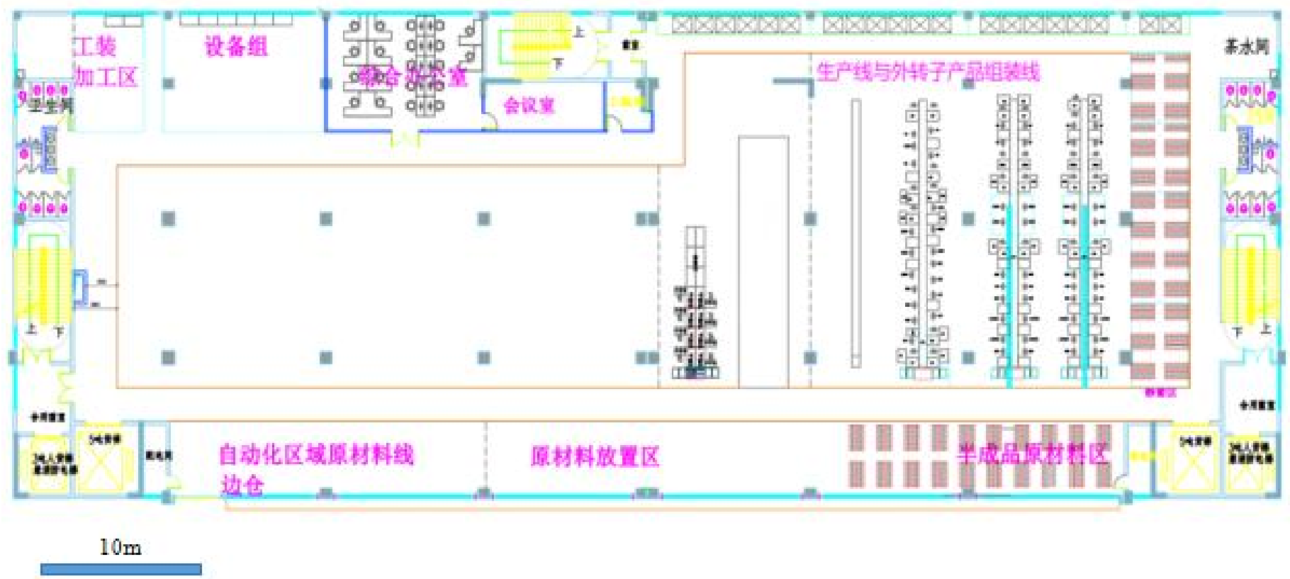
图 3-6 A 栋厂房车间平面布置图 (3 楼)
