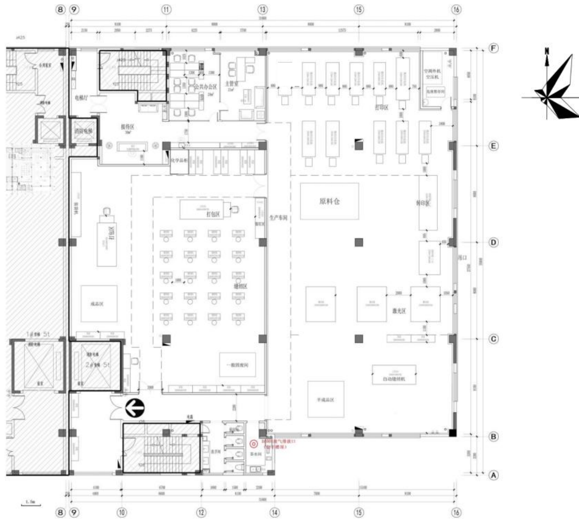
图 3-4 项目厂区平面图
