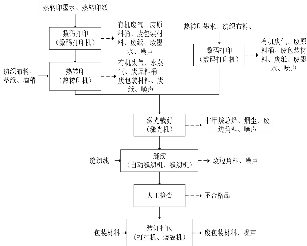
图 3-5 项目生产工艺流程图
