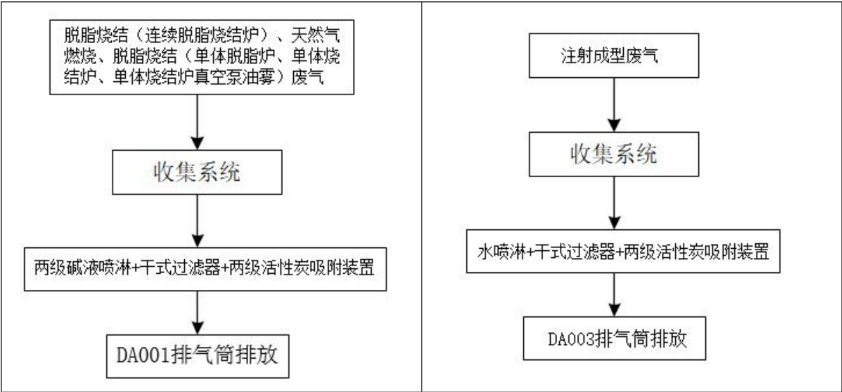
图 4-1 项目废气治理工艺流程图
