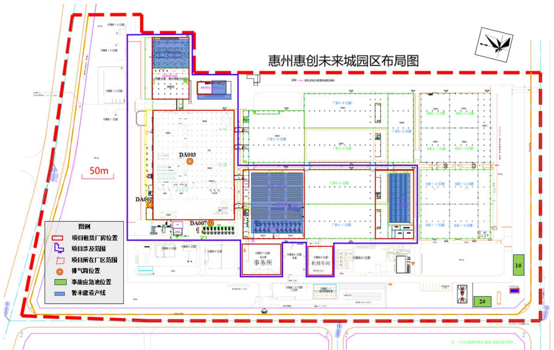
图 3-4 项目厂区总平面布置图
